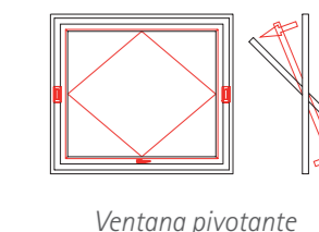
Ventana pivotante
