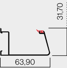
Colector de clipaje 050208
