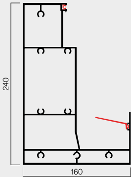
Viga P-240x160 mm 050618
