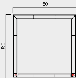
Columna abierta U 160x160 050610
